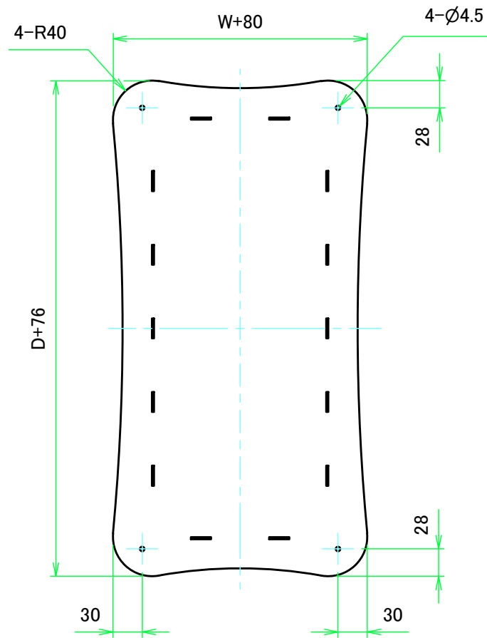
上カバー表面 / Top cover Frontside
